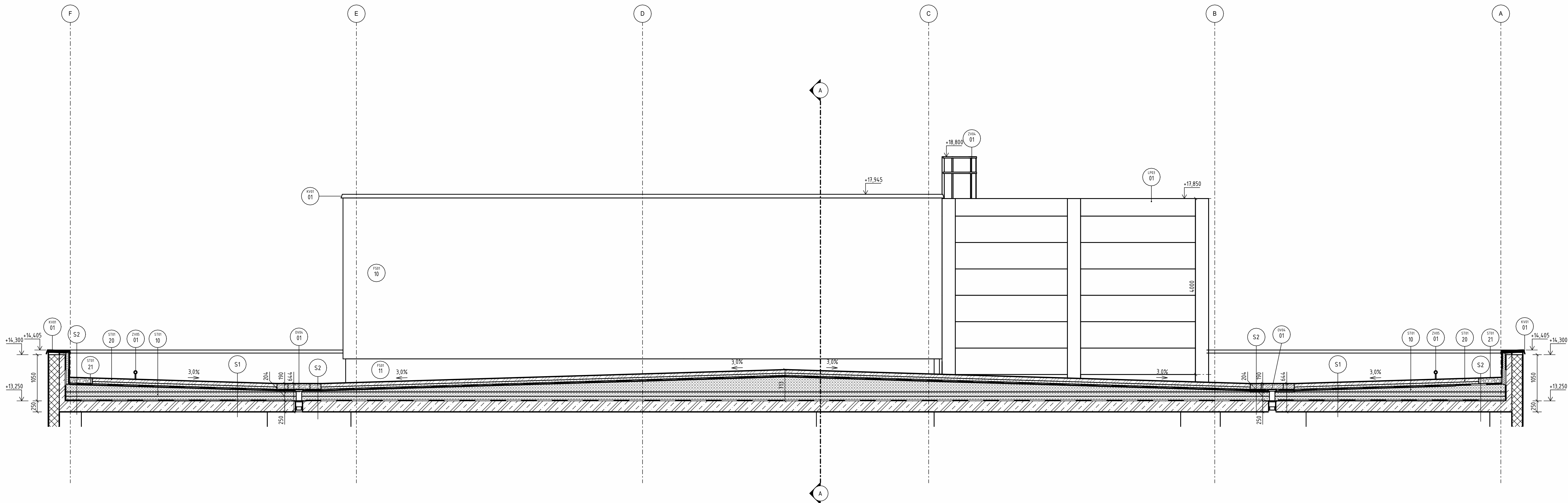
REZ C - POZDÍŽNY REZ STREŠNÝM PLÁŠŤOM
